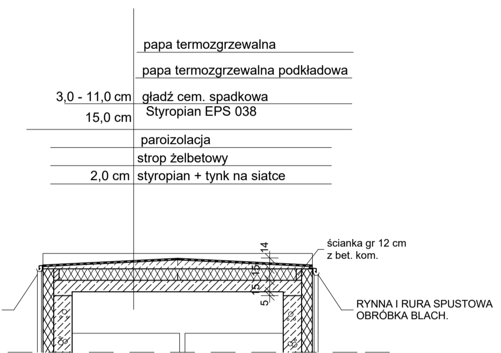
PRZEKRÓJ 3-3 - daszek przedsonka
